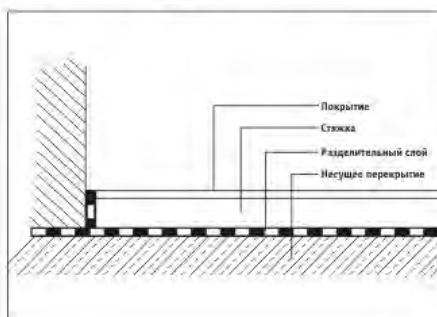
Рис.6 Стяжка на разделительном слое
