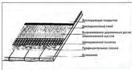
Рис.9 Укладка покрытия пола на старом деревянном дощатом полу; Выравнивание специальной шпаклевкой
