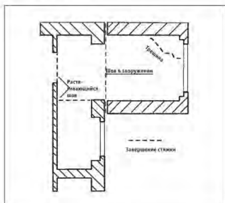
Рис.7 Швы в стяжке
