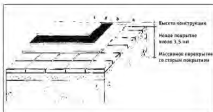
Рис.9 Эластичное покрытие пола на керамических плитках
