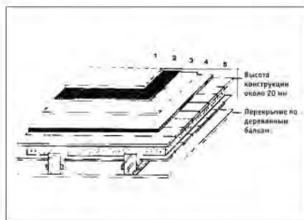
Рис.8 Укладка покрытия пола на старом деревянном дощатом полу; Выравнивание древесно-опилочными плитами
