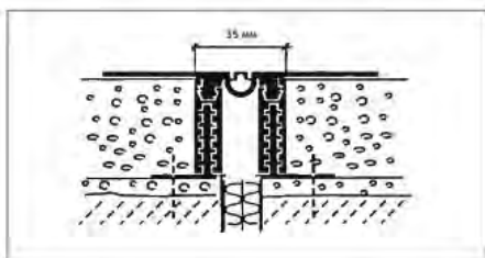
Рис.11 MIGUA - заделка деформационных осадочных швов Fr30
