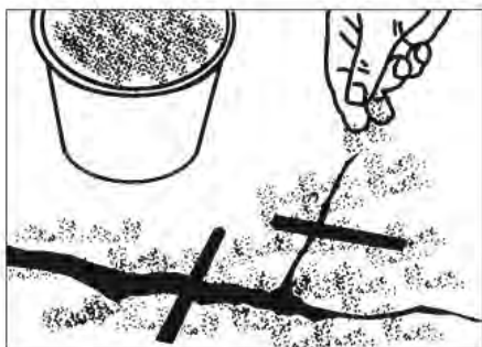
Рис. 3.5 Посыпание кварцевым песком с избытком
