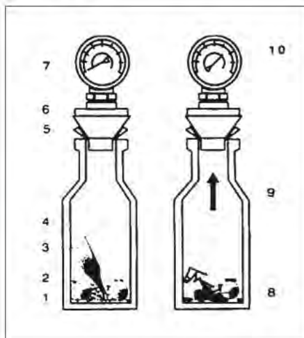
Рис. 4 Прибор СМ
